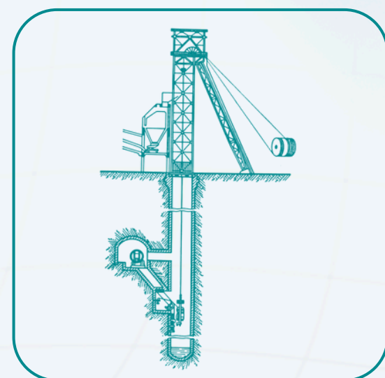
Скиповые машины
