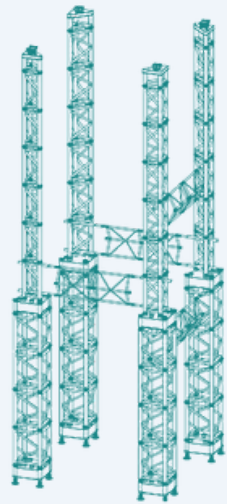
Несущая башенная система Greiner Power Tower •Г/п до 3600 т •Высота подъёма до 31 м
