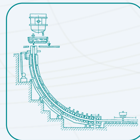
МНЛЗ
