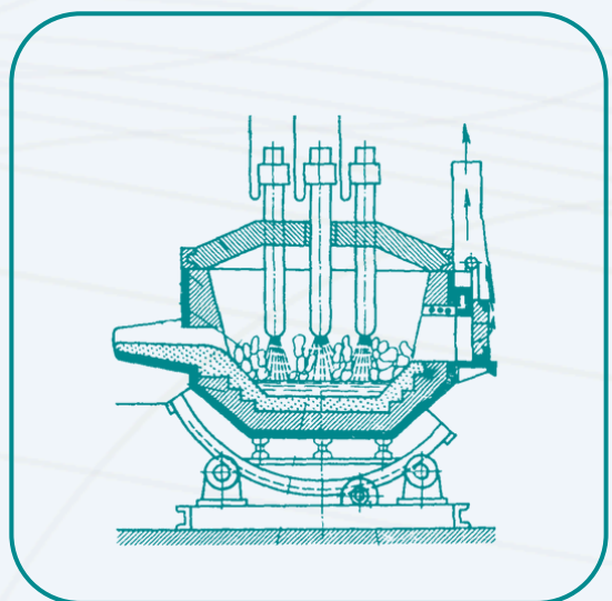
Печи
